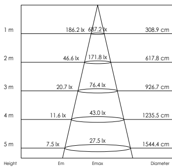
DIAGRAMMEN GEBASEERD OP 40004310 (215X215 MM / 3000K / 30W) DIAGRAMS BASED ON 40004310 (215X215 MM / 3000K / 30W)
